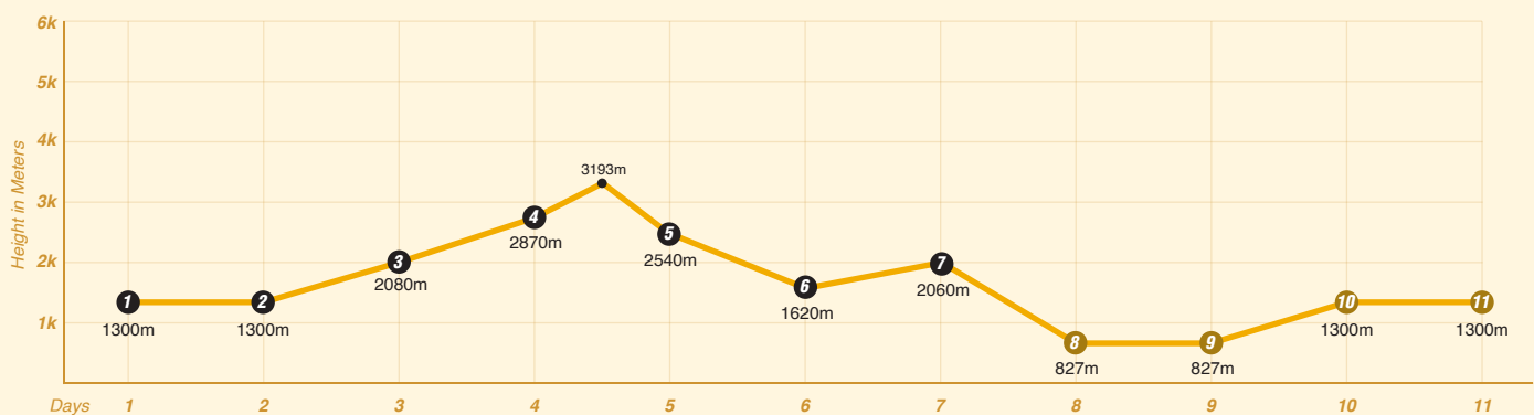
ALTITUDE CHART
